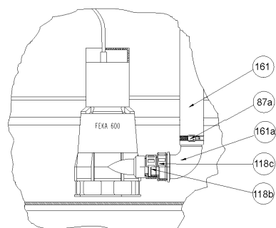
FEKA 600
