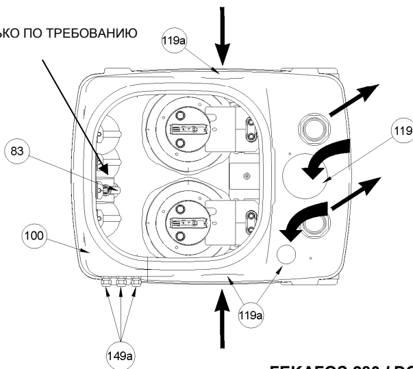
FEKAFOS 280 / DOUBLE
