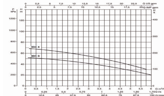
MICRA HS 304
