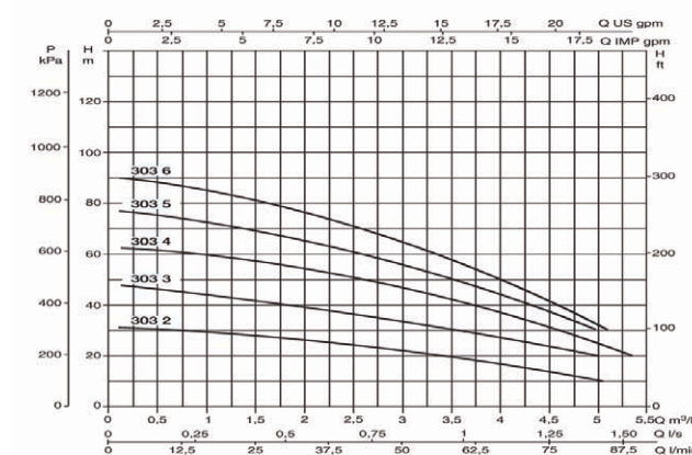
MICRA HS 303
